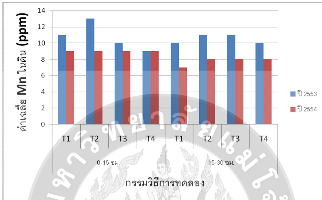
ภาพที่ 20 ผลการวิเคราะห์ค่า Mn ในดินที่ระดับความลึก 0-15 และ 15-30 เซนติเมตร
