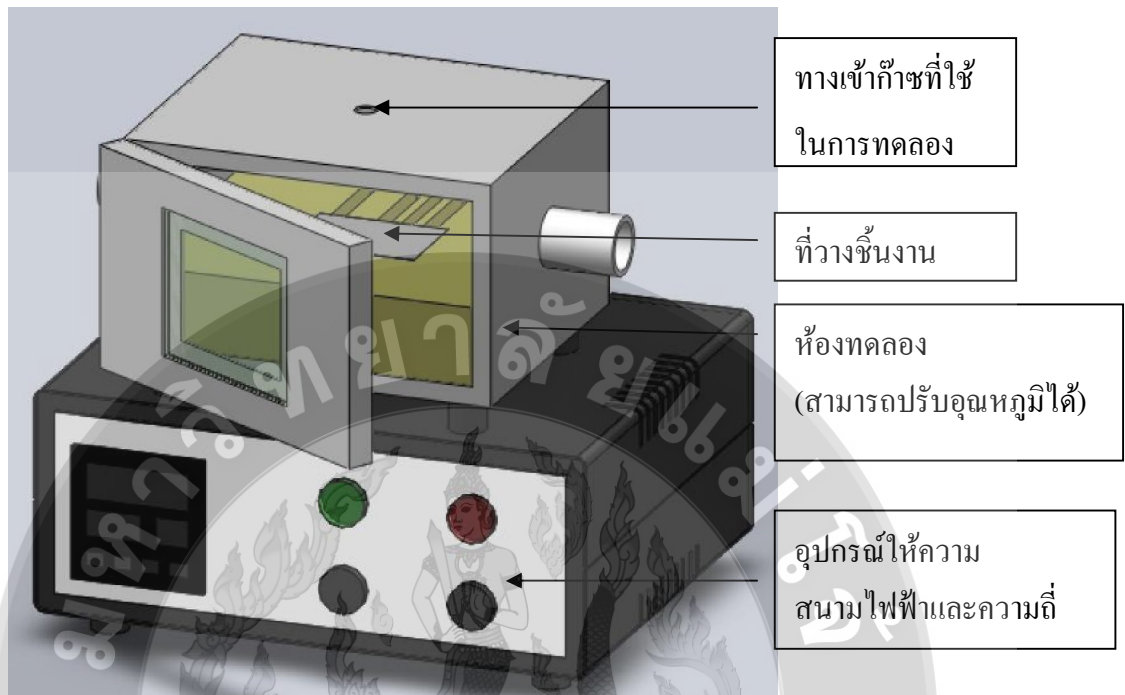
ภาพที่ 6 แสดงเครื่องกำเนิดโคล์พลาสมา
