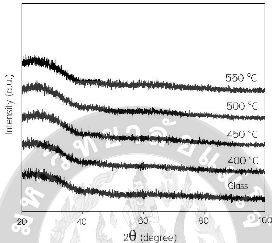
ภาพที่ 9 สเปกตรัมการเลี้ยวเบนของรังสีเอ็กซ์ของฟิล์มไทเทเนียมไดออกไซด์เอ็กซ์ (XRD) ของฟิล์มไทเทเนียมไดออกไซด์ไม่ได้อยู่ภายใต้สภาวะของไนโตรเจนพลาสมา มีการเพิ่มอุณหภูมิตั้งแต่ 400 องศาเซลเซียส ถึง 550 องศาเซลเซียส
