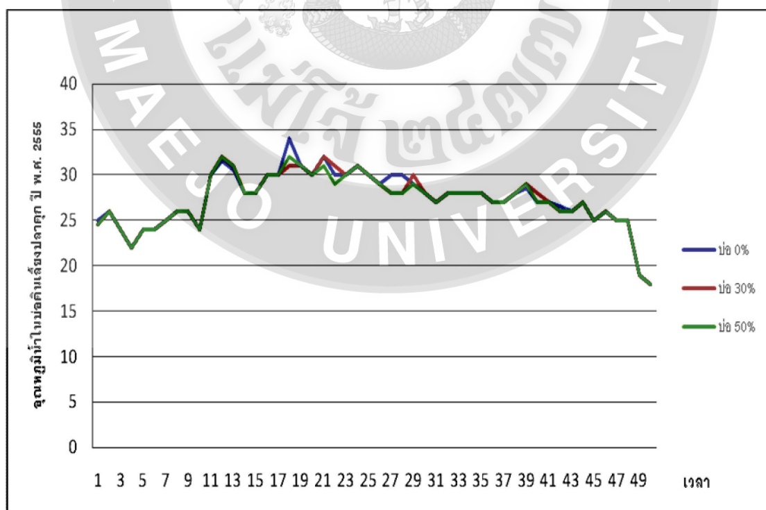
ภาพที่ 10 เปรียบเทียบการเปลี่ยนแปลงอุณหภูมิน้ำ( Water temperature ) ในบ่อดินเลี้ยงปลาคู ทั้งที่ใช้และไม่ใช้ระบบชีววิถีผักตบชวา ปี พ.ศ. 2555
