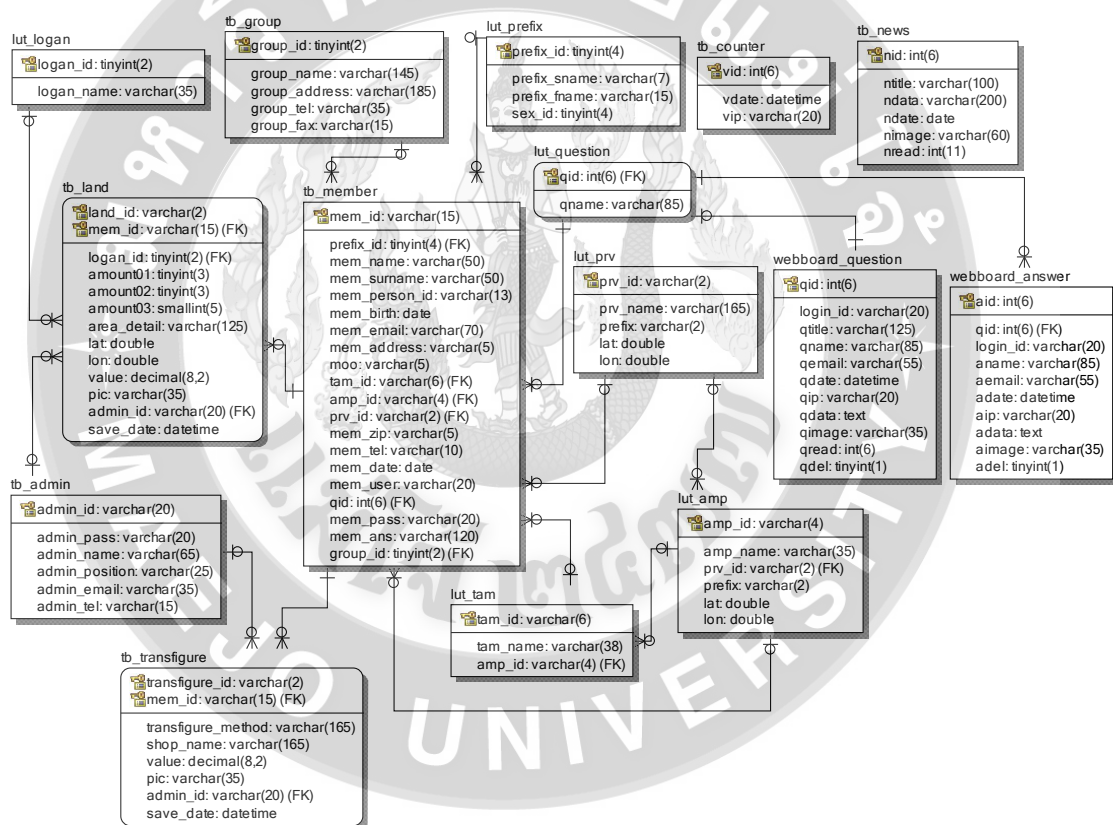
ภาพที่ 5 แผนภาพแสดงความสัมพันธ์ของข้อมูลของระบบฐานข้อมูลการจัดการธุรกิจ ค้าไฮอินทรีย์ในภาคเหนือตอนบน (E-R Diagram)
