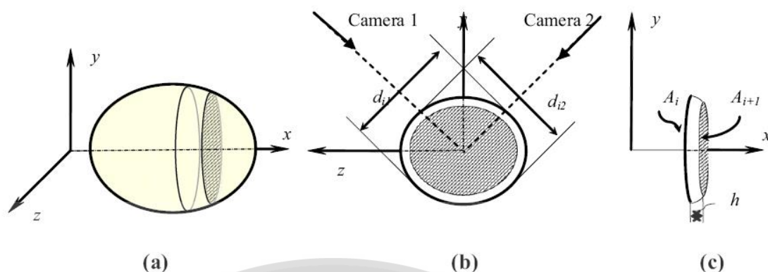
ภาพที่ 16 การแบ่งส่วนภาพเพื่อประมาณหาปริมาตรของผลไม้ (Omid, Khojastehnazhand and Tabatabaeefar, 2010)
