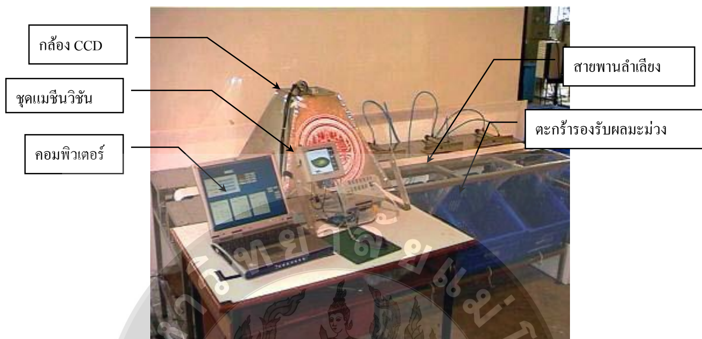
ภาพที่ 9 เครื่องคัดมะม่วงระบบแม่ชีนวิชัน
