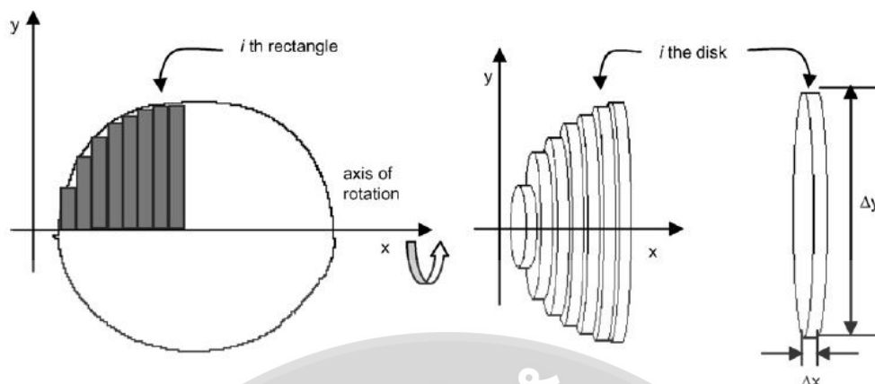
ภาพที่ 15 แผ่นกลมเสมือนสร้างขึ้นโดยโปรแกรมคอมพิวเตอร์เพื่อคำนวณหาปริมาตรของผลแดงโม (Koc, 2007)
