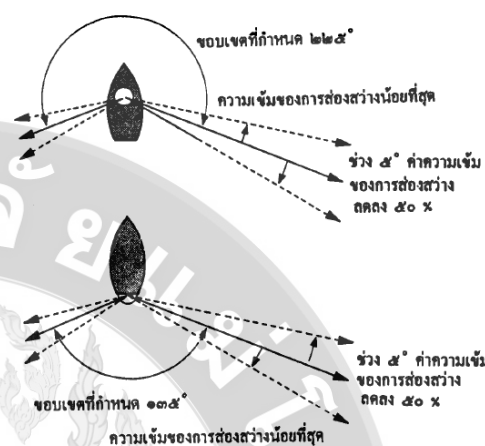
ภาพที่ 4.18 ขอบเขตการเห็นไฟของโคมไฟเสากระโดง
