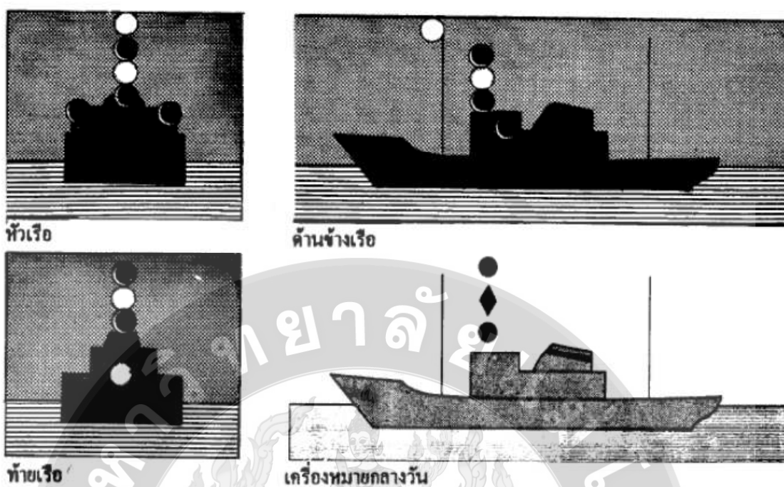
ภาพที่ 4.34 การใช้สัญญาณหมอกสำหรับเรือมีความยาวตั้งแต่ 50 เมตรขึ้นไป ไม่สามารถบังคับการเดินได้คล่องตัว ขณะเคลื่อนที่
