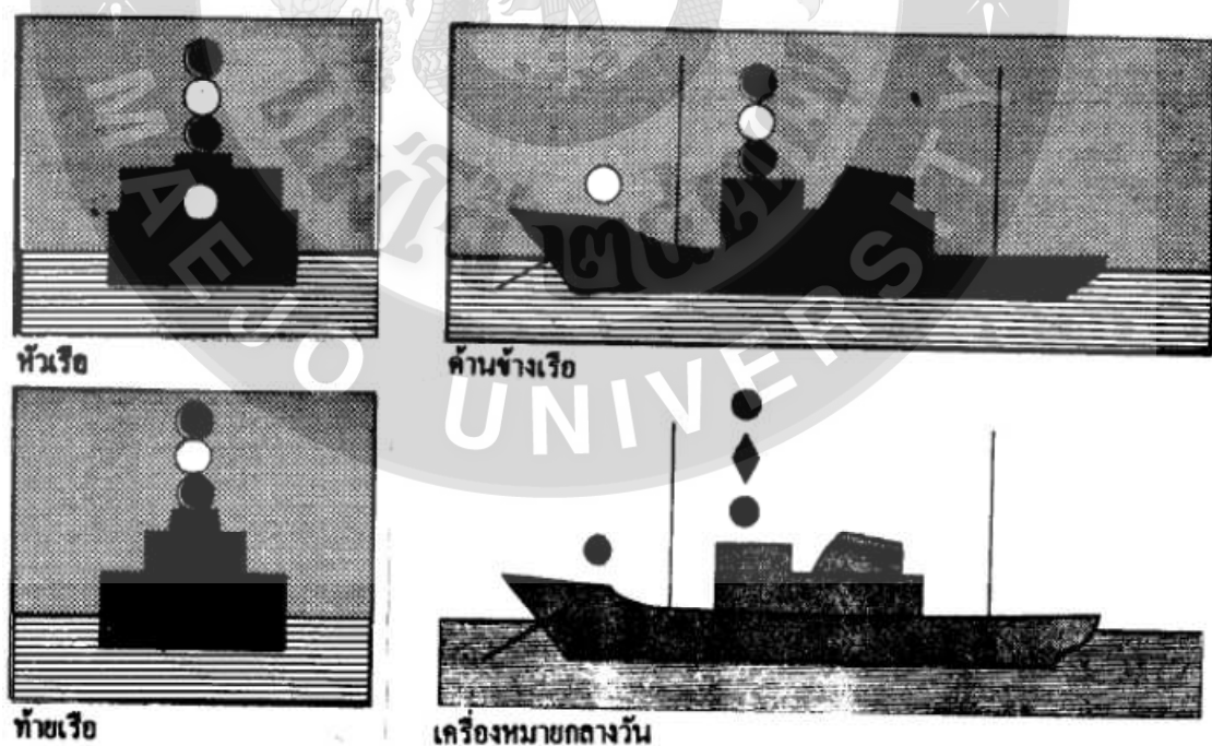
ภาพที่ 4.35 การใช้สัญญาณหมอกสำหรับเรือมีความยาวตั้งแต่ 50 เมตรขึ้นไป ไม่สามารถบังคับการเดินได้คล่องตัว ขณะจอดทอดสมอ
