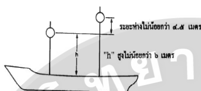
ภาพที่ 4.2 ความยาวของเรือตั้งแต่ 20 เมตร ขึ้นไป
