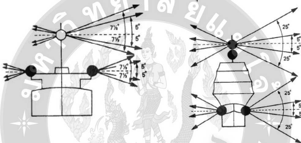
ภาพที่ 4.20 ขอบเขตการเห็นของโคมไฟในทางดิ่ง
