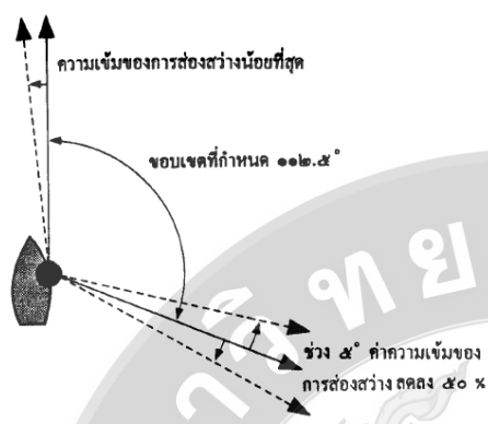
ภาพที่ 4.17 ขอบเขตการเห็นไฟของโคมไฟข้างเรือ
