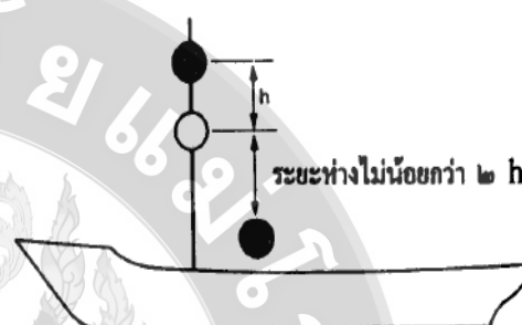
ภาพที่ 4.11 การติดตั้งโคมไฟความสูงของไฟที่เห็นได้รอบทิศทางสำหรับเรือประมงขณะทำการประมง
