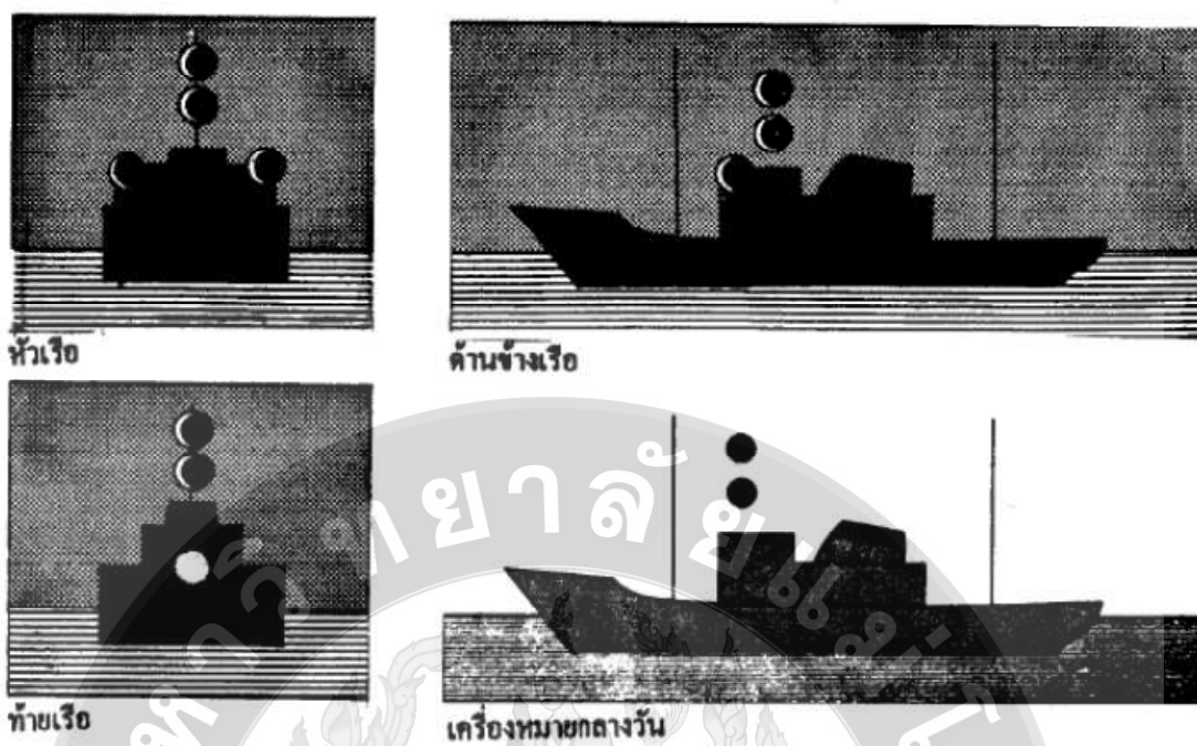
ภาพที่ 4.32 การใช้สัญญาณหมอกสำหรับเรือไม่อยู่ในบังคับ ขณะเคลื่อนที่
