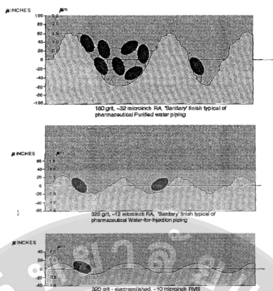
ภาพที่ 5 เปรียบเทียบการเกาะยึดของจุลินทรีย์บนวัสดุที่มีลักษณะพื้นผิวแตกต่างกัน ที่มา: สิทธิโชค (2547)
