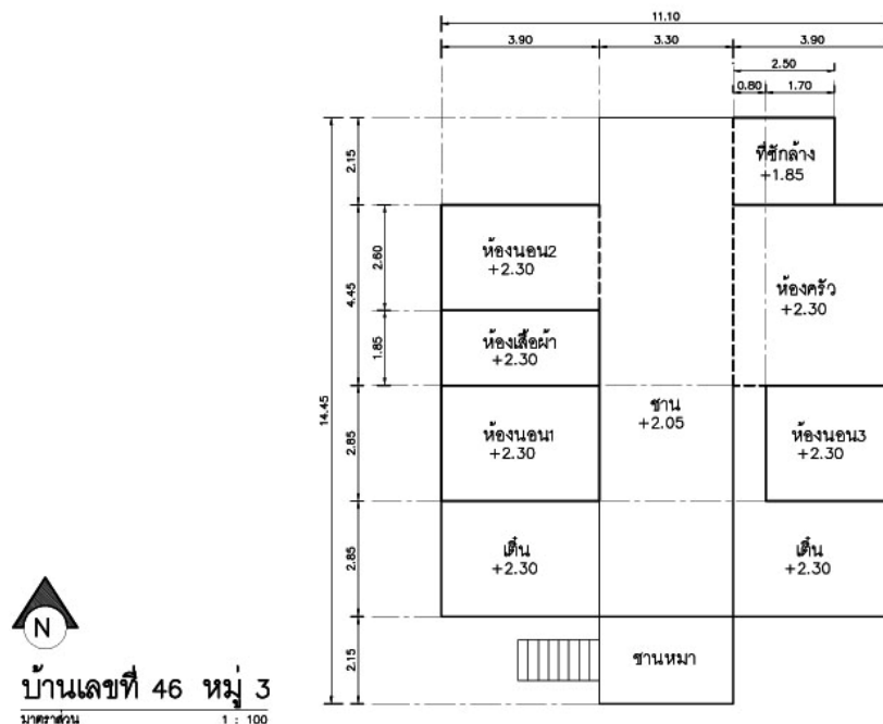
ภาพที่ 38 ผังพื้นที่อยู่อาศัยภายในเรือน
