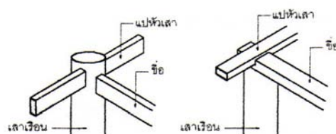
ภาพลายเส้นที่ 4 แสดงช่อ แป้นหัวเสา
