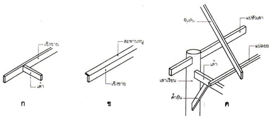
ภาพลายเส้นที่ 6 แสดงเชิงชาย เสา สะพานหนู แป้วลอย ค้ำยัน
