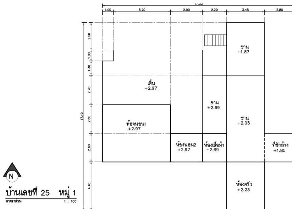
ภาพที่ 41 ผังพื้นที่ใช้สอยภายในเรือน
