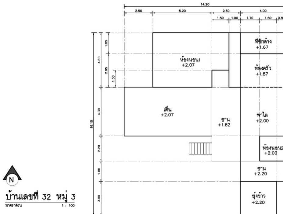
ภาพที่ 44 ผังพื้นการใช้สอยภายในเรือน
