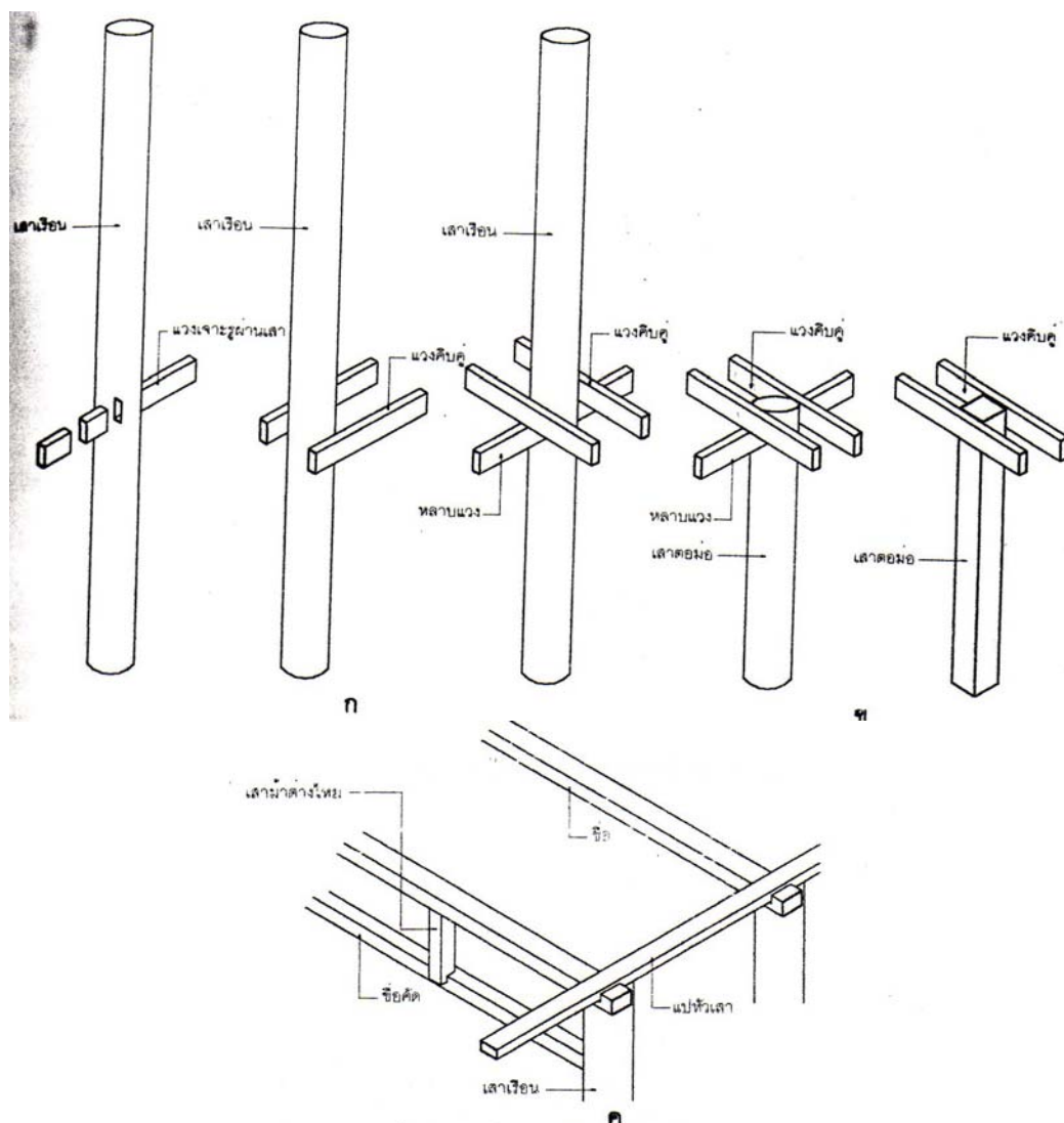
ภาพลายเส้นที่ 1 แสดงเสาริออนเสาคีมเสาคีมค้ำ เสาคีมค้ำค้ำ
