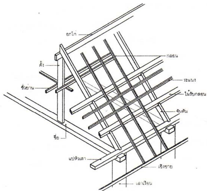
ภาพลายเส้นที่ 5 แสดงส่วนประกอบโครงสร้างหลังคา
