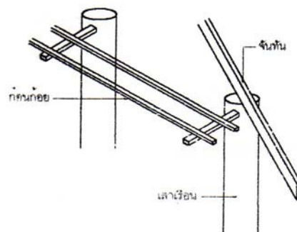
ภาพลายเส้นที่ 7 แสดงกันสาด
