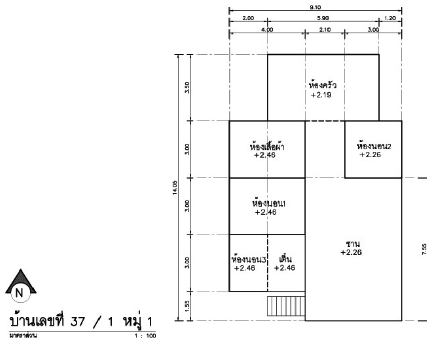
ภาพที่ 47 ผังพื้นที่ใช้สอยภายในเรือน
