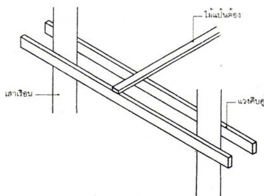
ภาพลายเส้นที่ 3 แสดงไม้แป้นตง
