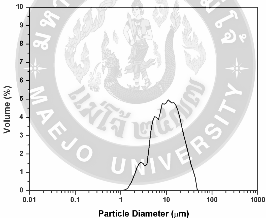
รูปที่ 4.1 แสดงการกระจายขนาดอนุภาคของจีเถ้าเคลือบด้วยเครื่อง particle size distribution
