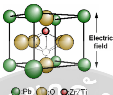
รูปที่ 2.3 ลักษณะโครงสร้างผลึกแบบเพอโรฟสไกต์ของเซรามิกเลเซอร์โคเนตไทเทเนต[4]
