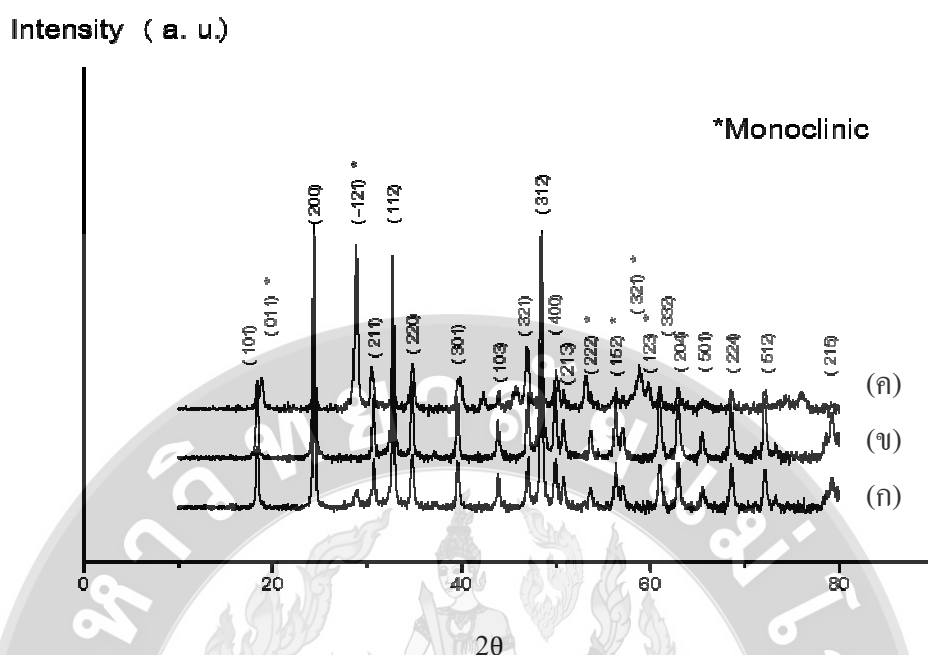
ภาพที่ 8 รูปแบบ XRD ของผงบิสมัธวานาเดตที่เตรียมโดยวิธีไมโครเวฟ ที่กำลังไฟฟ้า 800 วัตต์ เวลา (ก) 2 และ (ข) 6 นาที
