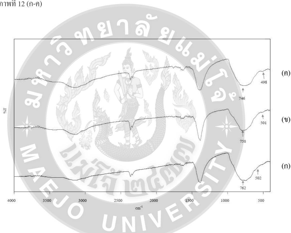
ภาพที่ 12 FTIR สเปกตรัมของผงบิสมัทวานาเดต ที่เตรียมโดยวิธีไมโครเวฟ กำลังไฟฟ้า 600 วัตต์ เวลา (ก) 2 นาที (ข) 4 นาที และ (ค) 6 นาที
