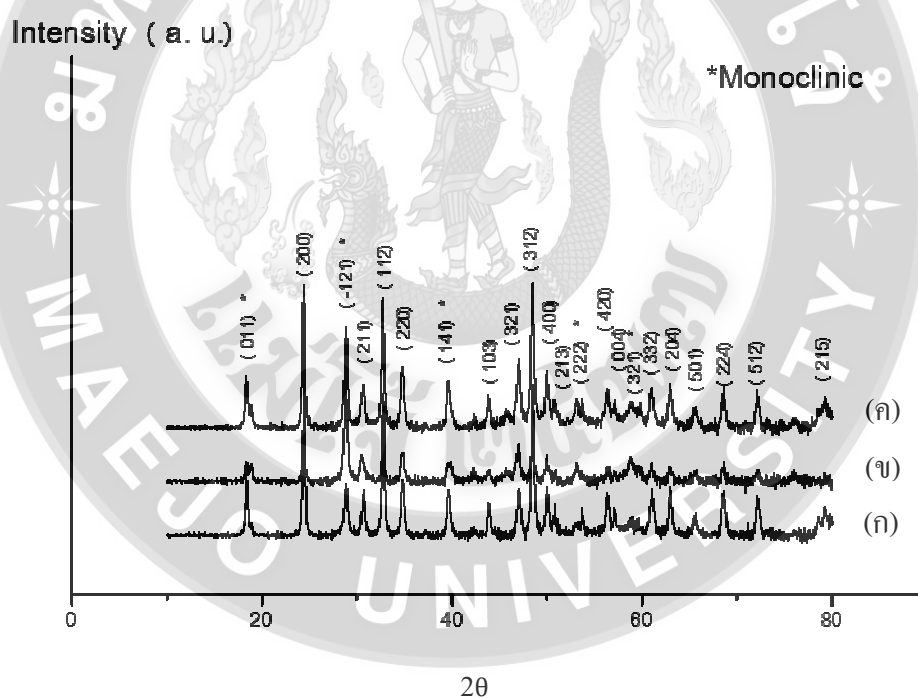
ภาพที่ 7 รูปแบบ XRD ของผงบิสมัทวานาเดตที่เตรียมโดยวิธีไมโครเวฟ ที่กำลังไฟฟ้า 700 วัตต์ เวลา (ก) 2 (ข) 4 นาที และ (ค) 6 นาที
