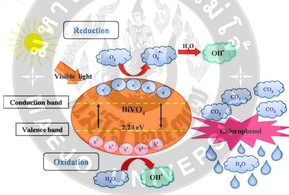
ภาพที่ 5 กลไกการกำจัดคลอโรฟีนอล ด้วยปฏิกิริยาโฟโตแคตาลิสต์ของบิสมัทวานาเดต ภายใต้การฉายแสงวิสิเบิล [34]
