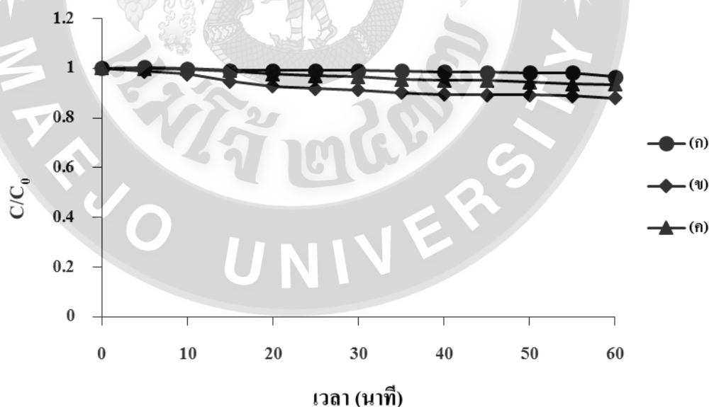
ภาพที่ 17 การสลายตัวของสารละลายเมทโรมิด โดยผงบิสมัธวานาเดตที่เตรียมโดยวิธีไมโครเวฟ กำลังไฟฟ้า 600 วัตต์ ที่เวลา (ก) ปราศจากผงบิสมัธวานาเดต (ข) 2 นาที และ (ค) 6 นาที
