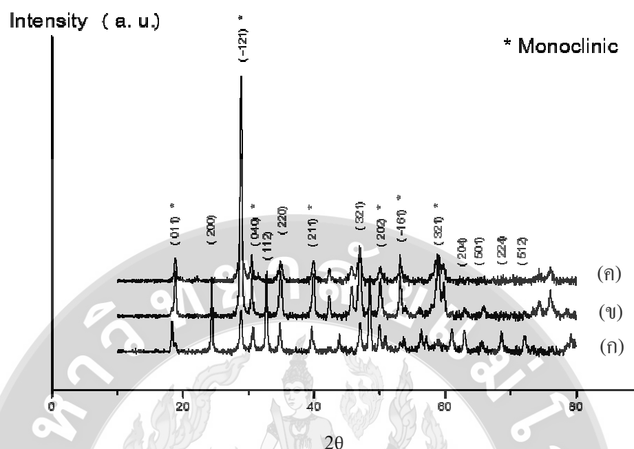
ภาพที่ 6 รูปแบบ XRD ของผงบิสมัธวานาเดตที่เตรียมโดยวิธีไมโครเวฟ ที่กำลังไฟฟ้า 600 วัตต์ เวลา (ก) 2 (ข) 4 นาที และ (ค) 6 นาที
