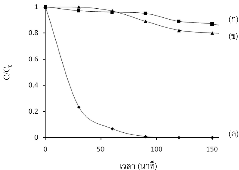
ภาพ 3.41 กราฟความสัมพันธ์ระหว่าง C/C_0 และเวลาของกระบวนการปฏิกิริยาโฟโตแคตตาไลติกส์ในการกำจัดฟีนอล โดยที่ (ก) ไม่เติมผงซิงค์ออกไซด์, (ข) ซิงค์ออกไซด์ที่เตรียมโดยวิธีตกตะกอนทางเคมี ทำการปรับค่าความเป็น กรด-ด่าง ของสารละลายผสมเท่ากับ 9 อุณหภูมิ 70 องศาเซลเซียส และ (ค) ซิงค์ออกไซด์มาตรฐาน
