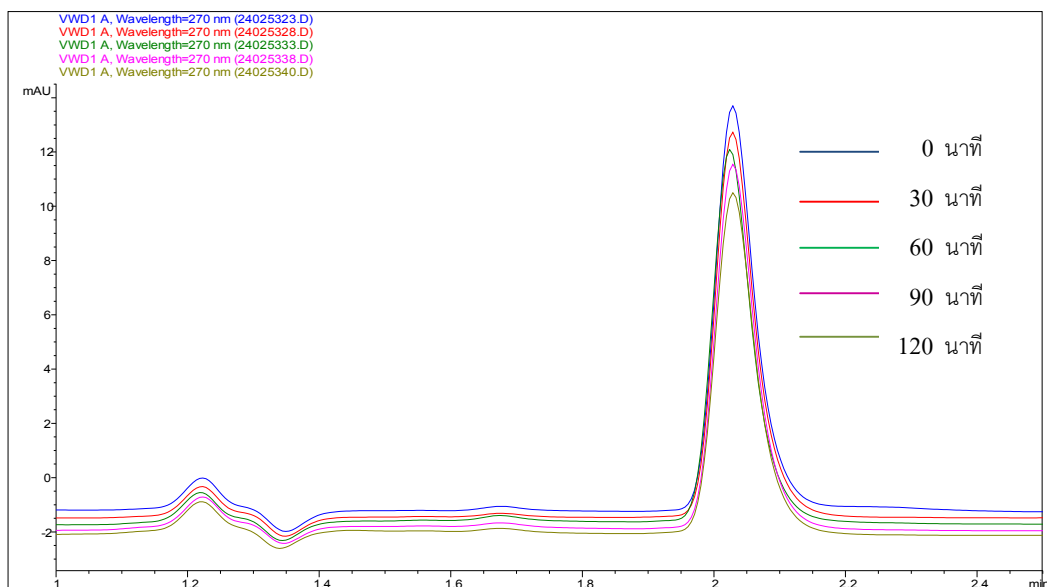
ภาพ 3.21 โคโรมาโทแกรมการสลายตัวของฟีนอล โดยผงไททาเนียมไดออกไซด์ ที่ได้จากการเตรียมโดยวิธีไฮโดรเทอร์มอล ที่อุณหภูมิ 80 องศาเซลเซียส เป็นเวลา 2 ชั่วโมง ปริมาตรฉีด 20 ไมโครลิตร โดยเครื่องโครมาโทกราฟของเหลวสมรรถนะสูง ที่ความยาวคลื่นของการตรวจวัดเท่ากับ 270 นาโนเมตร
