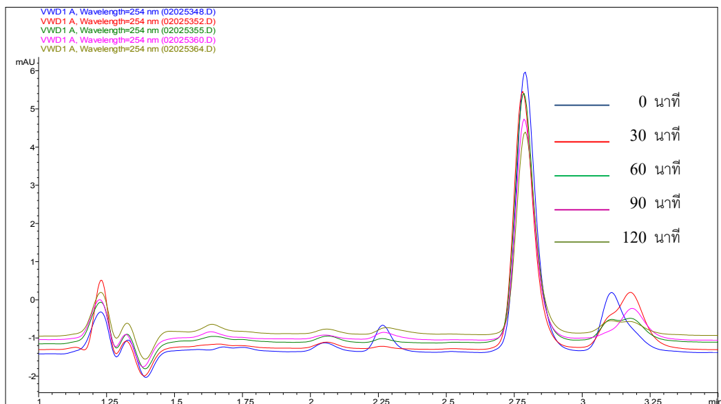
ภาพ 3.26 โครมาโทแกรมการสลายตัวของ 2-คลอโรฟีนอล โดยผงไททาเนียมไดออกไซด์ ที่ได้จากการเตรียมโดยวิธีไฮโดรเทอร์มอล ที่อุณหภูมิ 80 องศาเซลเซียส เป็นเวลา 2 ชั่วโมง ปริมาตรฉีด 20 ไมโครลิตร โดยเครื่องโครมาโทกราฟของเหลวสมรรถนะสูง ที่ความยาวคลื่นของการตรวจวัดเท่ากับ 254 นาโนเมตร
