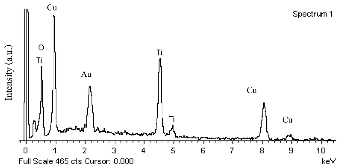
ภาพ 3.12 EDS ของผงไททาเนียมไดออกไซด์ ที่ได้จากการสังเคราะห์โดยวิธีไฮโดรเทอร์มอล ที่อุณหภูมิ 100 องศาเซลเซียส เป็นเวลา 6 ชั่วโมง
