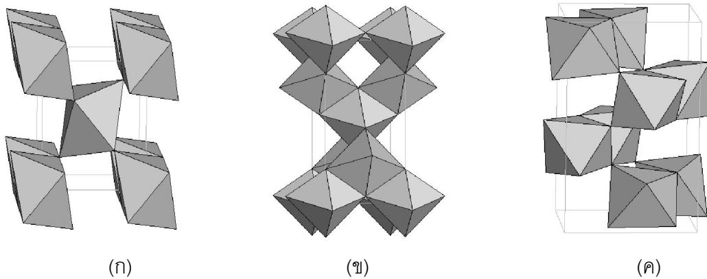
ภาพ 1.4 โครงสร้างของไททาเนียมไดออกไซด์ (ก) แบบรูไทล์ (ข) แบบอนาเทส
