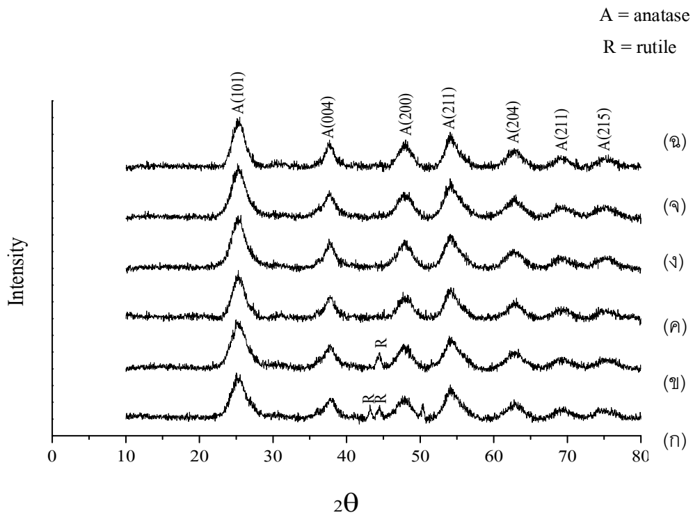
ภาพ 3.2 รูปแบบ XRD ของผงไททาเนียมไดออกไซด์ ที่เตรียมโดยวิธีไฮโดรเทอร์มอล ที่อุณหภูมิ (ก) 80 องศาเซลเซียส เป็นเวลา 2 ชั่วโมง (ง) 100 องศาเซลเซียส เป็นเวลา 2 ชั่วโมง (ข) 80 องศาเซลเซียส เป็นเวลา 4 ชั่วโมง (จ) 100 องศาเซลเซียส เป็นเวลา 4 ชั่วโมง (ค) 80 องศาเซลเซียส เป็นเวลา 6 ชั่วโมง (ฉ) 100 องศาเซลเซียส เป็นเวลา 6 ชั่วโมง
