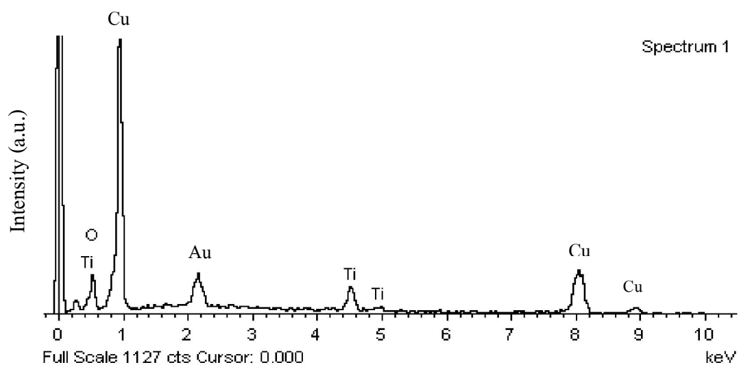
ภาพ 3.11 EDS ของผงไททาเนียมไดออกไซด์ ที่ได้จากการสังเคราะห์โดย วิธีไฮโดรเทอร์มอล ที่อุณหภูมิ 100 องศาเซลเซียส เป็นเวลา 4 ชั่วโมง
