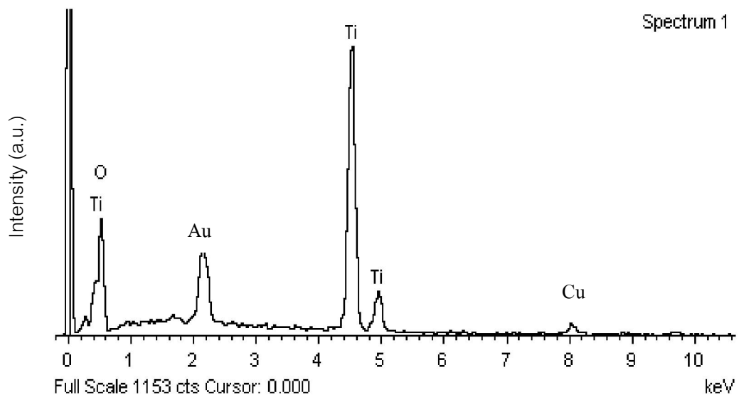
ภาพ 3.6 EDS ของผงไททาเนียมไดออกไซด์มาตรฐาน
