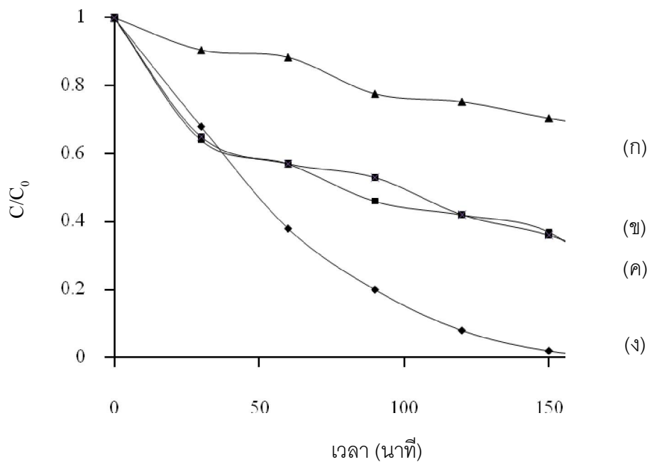
ภาพ 3.50 กราฟความสัมพันธ์ระหว่าง C/C_0 และเวลาของกระบวนการปฏิกิริยาโฟโตแคตาไลติกส์ในการกำจัด 2,4 ไดคลอโรฟีนอล โดยที่ (ก) ไม่เติมผงซิงค์ออกไซด์, (ข) ผงซิงค์ออกไซด์ที่ได้จากการเตรียมโดยวิธีไฮโดรเทอร์มอล ที่อุณหภูมิ 100 องศาเซลเซียส เป็นเวลา 4 ชั่วโมง, (ค) ผงซิงค์ออกไซด์ที่เตรียมโดยวิธีตกตะกอนทางเคมี ทำการปรับค่าความเป็นกรด-ด่างของสารละลายผสมเท่ากับ 9 ที่อุณหภูมิ 70 องศาเซลเซียส และ (ง) ผงซิงค์ออกไซด์มาตรฐาน
