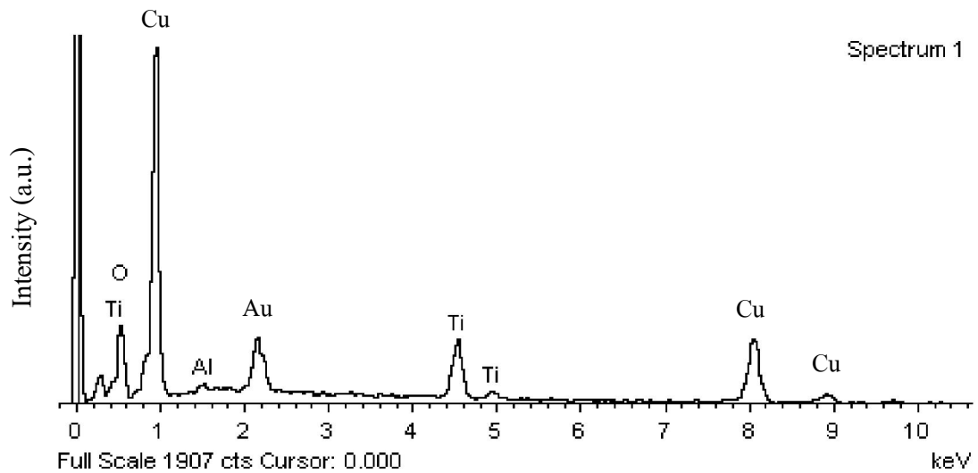
ภาพ 3.8 EDS ของผงไททาเนียมไดออกไซด์ ที่ได้จากการสังเคราะห์โดยวิธีไฮโดรเทอร์มอล ที่อุณหภูมิ 80 องศาเซลเซียส เป็นเวลา 4 ชั่วโมง
