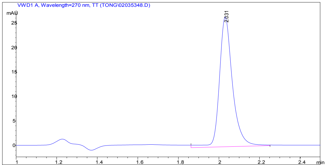
ภาพ 3.14 โครมาโทแกรมของสารละลายมาตรฐานฟีนอล เข้มข้น 5 มิลลิกรัมต่อลิตร ปริมาตรฉีด 20 ไมโครลิตร โดยเครื่องโครมาโทกราฟของเหลวสมรรถนะสูง ที่ความยาวคลื่นของการตรวจวัดเท่ากับ 270 นาโนเมตร
