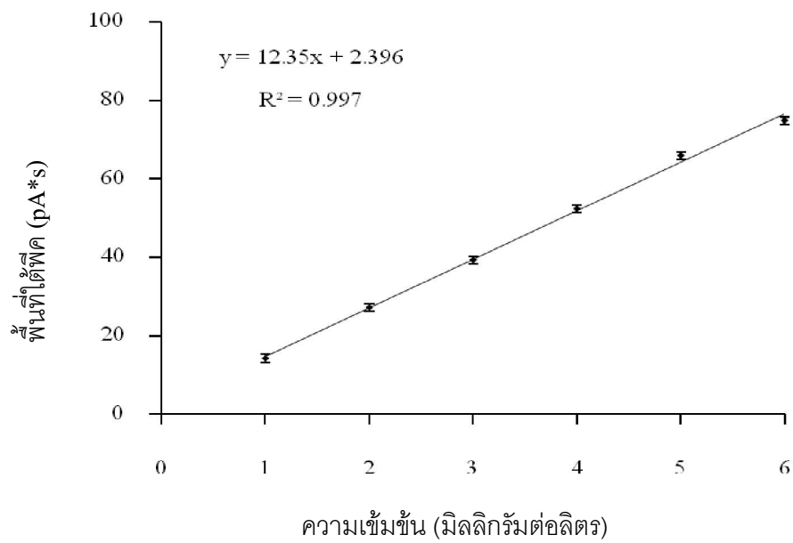
ภาพ 3.15 กราฟมาตรฐานของสารละลายมาตรฐาน 2-คลอโรฟีนอล
