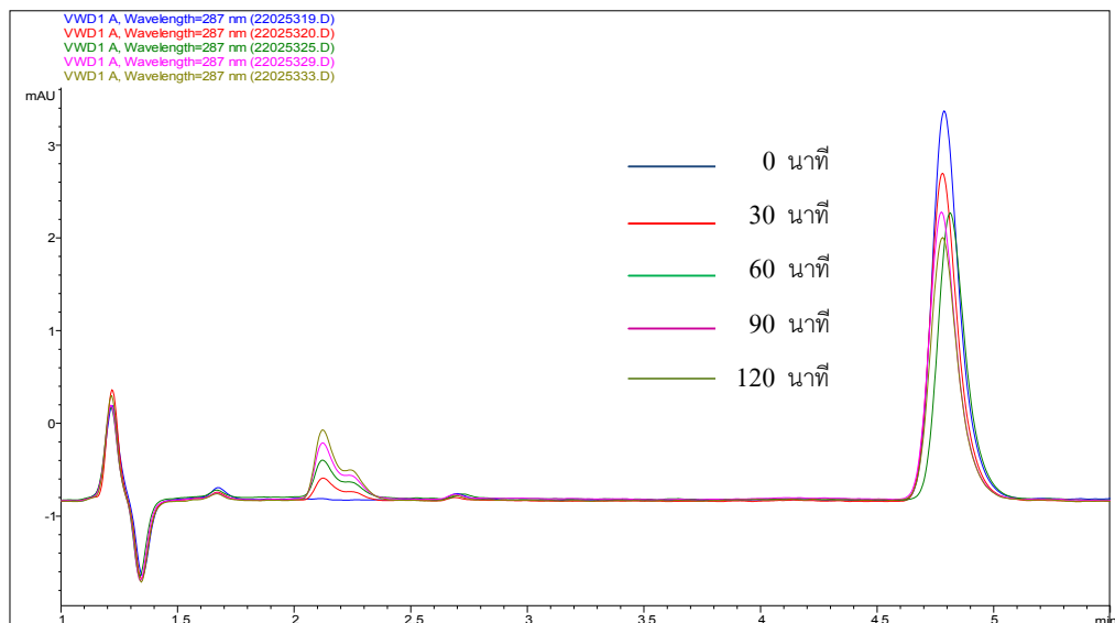
ภาพ 3.31 โครมาโทแกรมการสลายตัวของ 2,4-ไดคลอโรฟีนอล โดยผงไททาเนียมไดออกไซด์ที่ได้จากการเตรียม โดยวิธีไฮโดรเทอร์มอล ที่อุณหภูมิ 80 องศาเซลเซียส เป็นเวลา 2 ชั่วโมง ปริมาตรฉีด 20 ไมโครลิตร โดยเครื่องโครมาโทกราฟของเหลวสมรรถนะสูง ที่ความยาวคลื่นของการตรวจวัดเท่ากับ 287 นาโนเมตร
