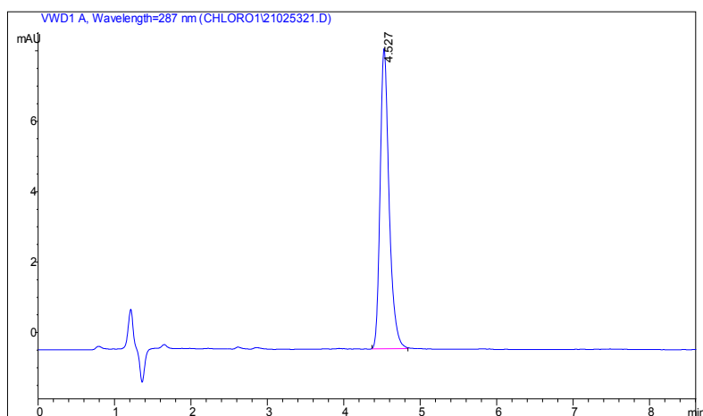
ภาพ 3.47 โครมาโทแกรมของสารละลายมาตรฐาน 2,4-ไดคลอโรฟีนอล เข้มข้น 5 มิลลิกรัมต่อลิตร ปริมาตรฉีด 20 ไมโครลิตร โดยเครื่องโครมาโทกราฟของเหลวสมรรถนะสูง ที่ความยาวคลื่นของการตรวจวัดเท่ากับ 287 นาโนเมตร
