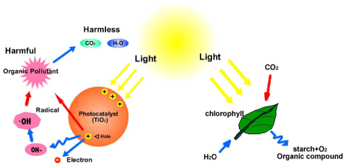
ภาพ 1.6 ปฏิกริยาโฟโตแคตาไลติกส์และโฟโตเคมี
