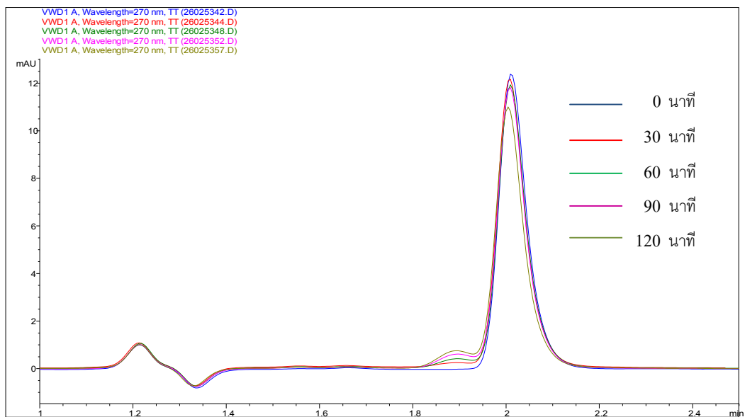
ภาพ 3.19 โครมาโทแกรมการสลายตัวของฟีนอลที่ปราศจากผงไททาเนียมไดออกไซด์ ปริมาตรฉีด 20 ไมโครลิตร โดยเครื่องโครมาโทกราฟของเหลวสมรรถนะสูง ที่ความยาวคลื่นของการตรวจวัดเท่ากับ 270 นาโนเมตร
