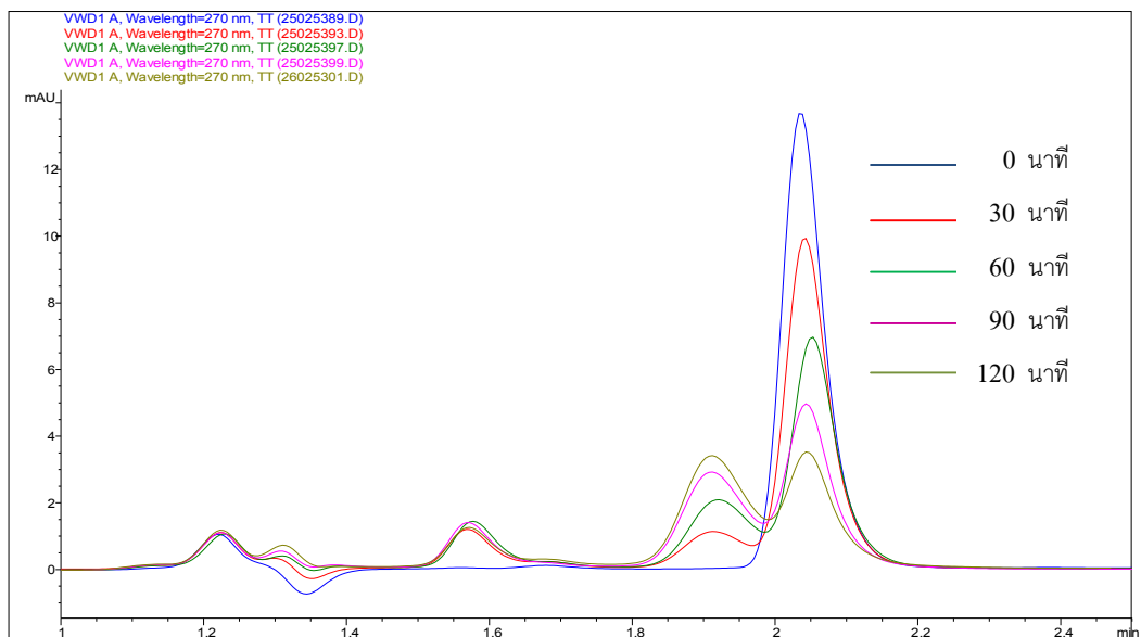
ภาพ 3.20 โครมาโทแกรมการสลายตัวของฟีนอล โดยผงไททาเนียมไดออกไซด์มาตรฐาน ปริมาตรฉีด ไมโครลิตร โดยเครื่องโครมาโทกราฟของเหลวสมรรถนะสูง ที่ความยาวคลื่นของการ ตรวจวัดเท่ากับ 270 นาโนเมตร
