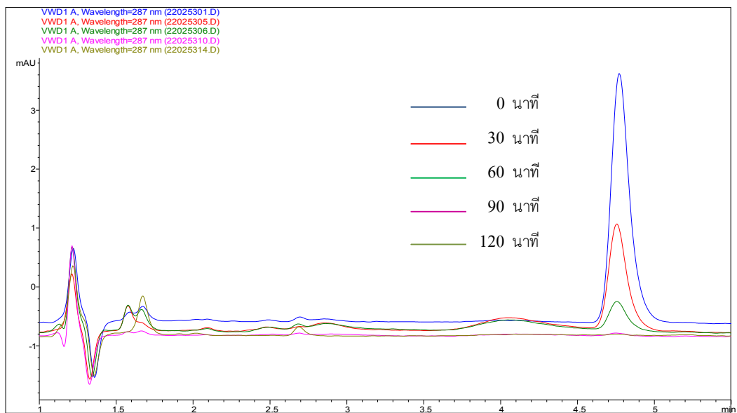
ภาพ 3.30 โครมาโทแกรมการสลายตัวของ 2,4-ไดคลอโรฟีนอล โดยผงไททาเนียมไดออกไซด์มาตรฐาน ปริมาตรฉีด 20 ไมโครลิตร โดยเครื่องโครมาโทกราฟของเหลวสมรรถนะสูงที่ความยาวคลื่นของการตรวจวัดเท่ากับ 287 นาโนเมตร
