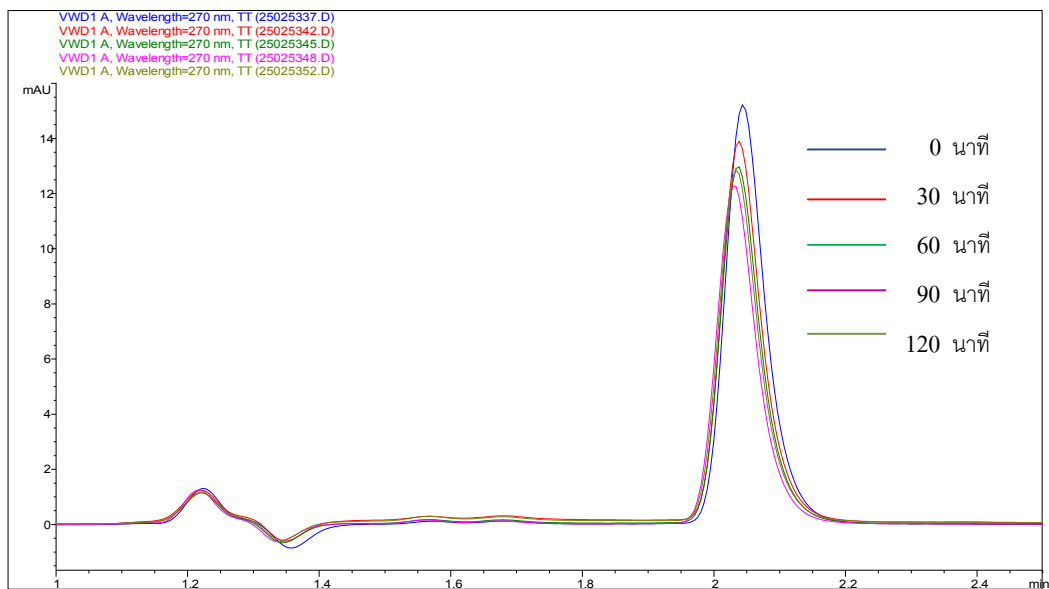
ภาพ 3.22 โคโรมาโทแกรมการสลายตัวของฟีนอล โดยผงไททาเนียมไดออกไซด์ ที่ได้จากการเตรียมโดยวิธีไฮโดรเทอร์มอล ที่อุณหภูมิ 100 องศาเซลเซียส เป็นเวลา 2 ชั่วโมง ปริมาตรฉีด 20 ไมโครลิตร โดยเครื่องโครมาโทกราฟของเหลวสมรรถนะสูง ที่ความยาวคลื่นของการตรวจวัดเท่ากับ 270 นาโนเมตร
