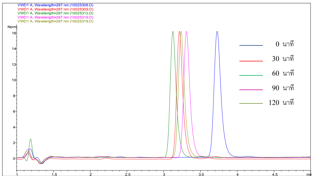
ภาพ 3.29 โครมาโทแกรมการสลายตัวของ 2,4-ไดคลอโรฟีนอลที่ปราศจากผงไททาเนียมไดออกไซด์ ปริมาตรฉีด 20 ไมโครลิตร โดยเครื่องโครมาโทกราฟของเหลวสมรรถนะสูง ที่ความยาวคลื่นของการตรวจวัดเท่ากับ 287 นาโนเมตร
