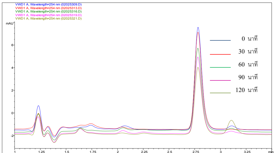
ภาพ 3.27 โครมาโทแกรมการสลายตัวของ 2-คลอโรฟีนอล โดยผงไททาเนียมไดออกไซด์ ที่ได้จากการเตรียมโดยวิธีไฮโดรเทอร์มอล ที่อุณหภูมิ 100 องศาเซลเซียส เป็นเวลา 2 ชั่วโมง ปริมาตรฉีด 20 ไมโครลิตร โดยเครื่องโครมาโทกราฟของเหลวสมรรถนะสูง ที่ความยาวคลื่นของการตรวจวัดเท่ากับ 254 นาโนเมตร
