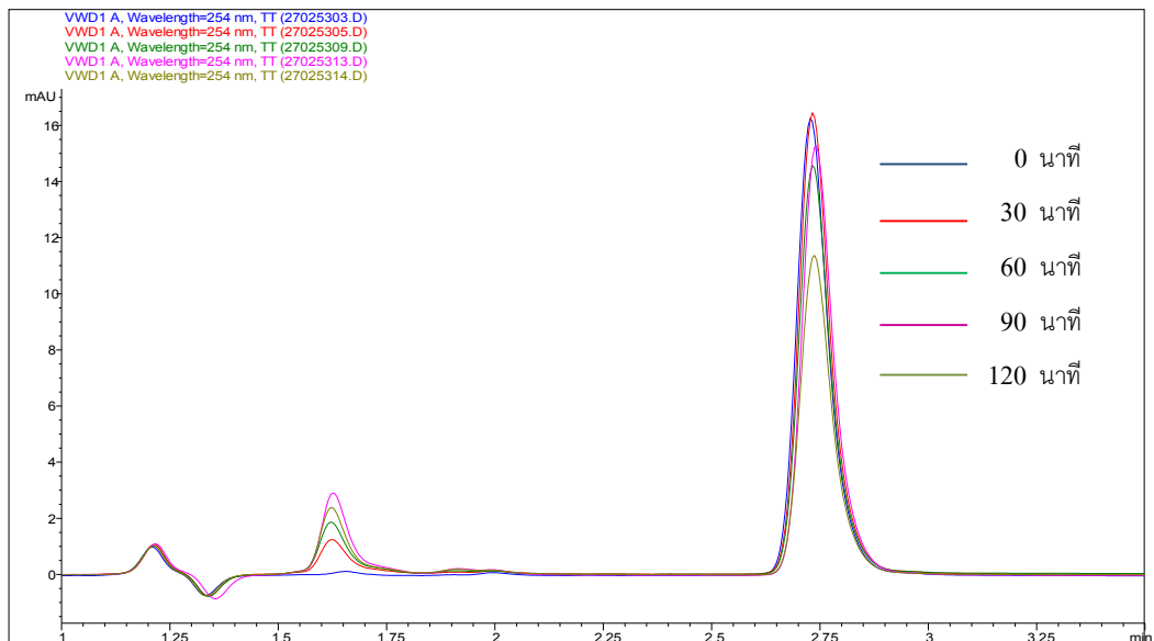
ภาพ 3.24 โคโรมาโทแกรมการสลายตัวของ 2-คลอโรฟีนอลที่ปราศจากผงไททาเนียมไดออกไซด์ ปริมาตรฉีด 20 ไมโครลิตร โดยเครื่องโครมาโทกราฟของเหลวสมรรถนะสูง ที่ความยาวคลื่นของการตรวจวัดเท่ากับ 254 นาโนเมตร
