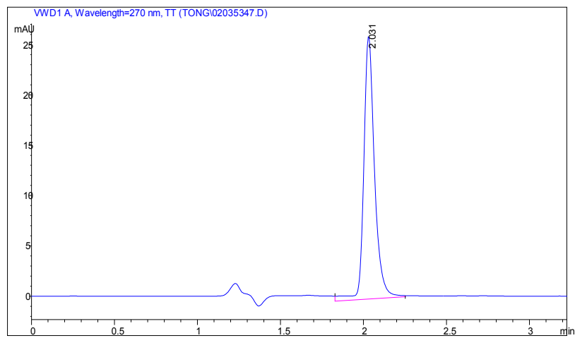
ภาพ 3.43 โคโรมาโทแกรมของสารละลายมาตรฐานฟีนอล เข้มข้น 5 มิลลิกรัมต่อลิตร ปริมาตรฉีด 20 ไมโครลิตร ความยาวคลื่นของการตรวจวัดเท่ากับ 270 นาโนเมตร
