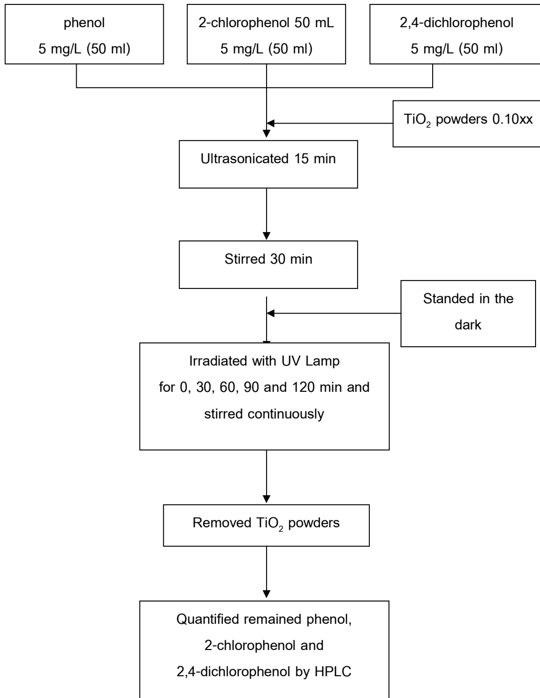
ภาพ 2.2 แผนผังการปฏิกิริยาโฟโตแคตาไลติกส์ ของผงไททาเนียมไดออกไซด์ที่เตรียม โดยวิธีไฮโดรเทอร์มอล
