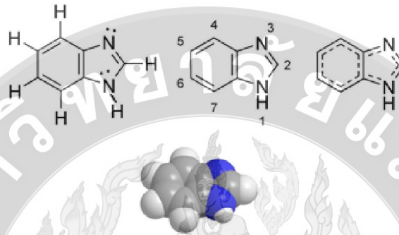
ภาพที่ 1 โครงสร้างเบนซิมิดาโซล
