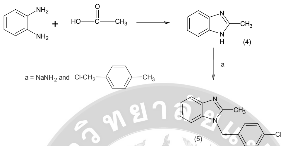
ภาพที่ 3 การสังเคราะห์สารคลอไมดาโซล
