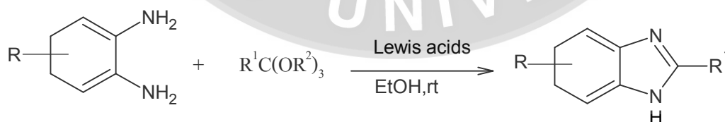
ภาพที่ 9 การสังเคราะห์เบนซิมิดาโซลโดยวิธีของ Zhan-Hui Zhang และคณะ
