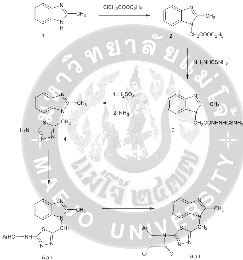
ภาพที่ 10 การสังเคราะห์ azetidin-2-ones
